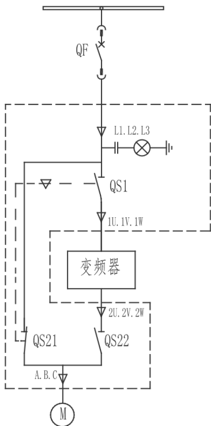
图3.23 手动旁路柜一次图
