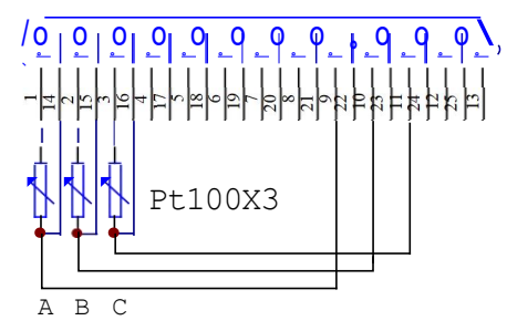
D/E/F型三路插头内部示意图
