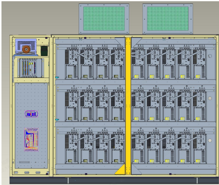
图3.18 典型单元柜排布图
