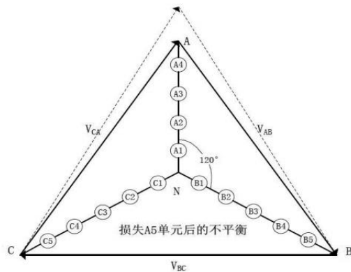
图6.6 A5单元旁路示意图
