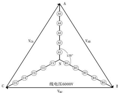
图6.5 5级变频器无旁路示意图
