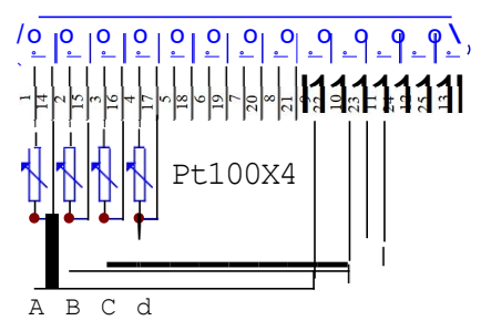
G/I型四路插头内部示意图
