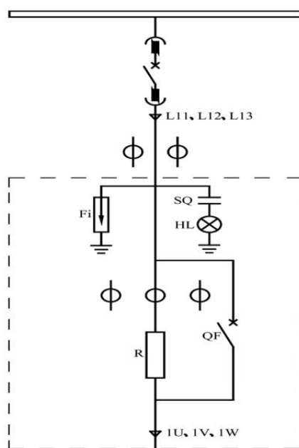
图 3.22 启动柜一次图
