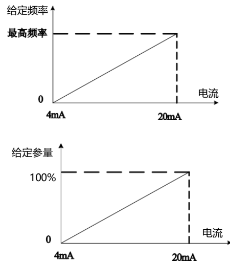
图5.22 模拟给定
