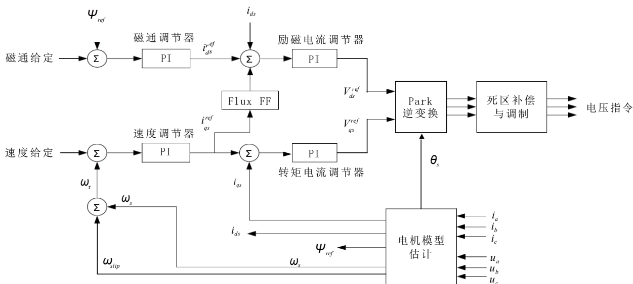
图6.8 异步机开环矢量控制框图
