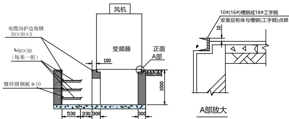
图7.6 电缆沟
