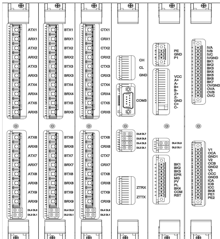
图3.6 控制器面板示意图
