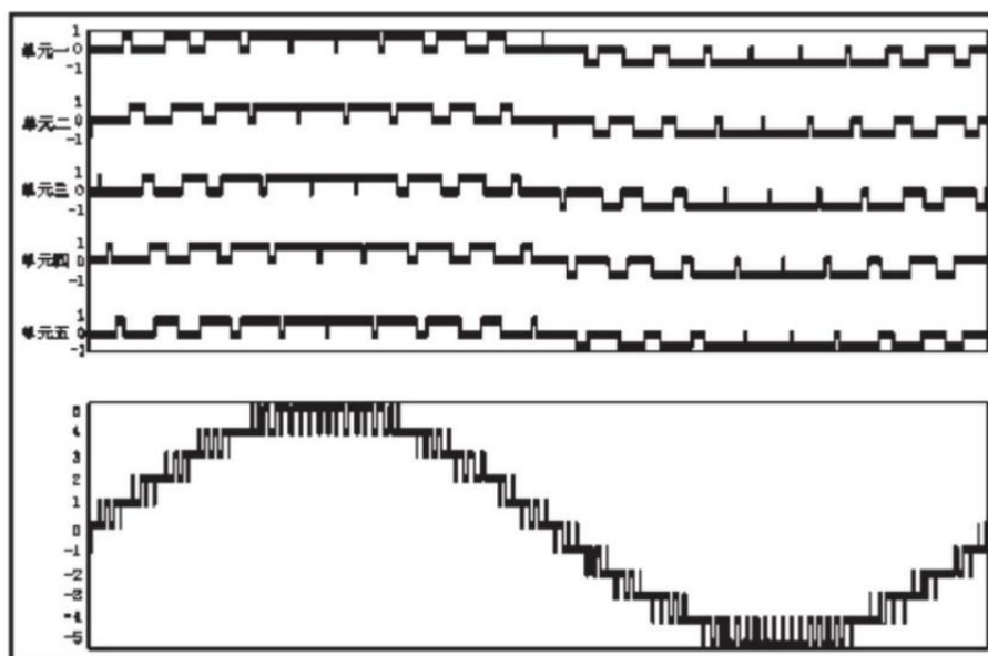
图3.5 6kV变频器输出相电压波形
