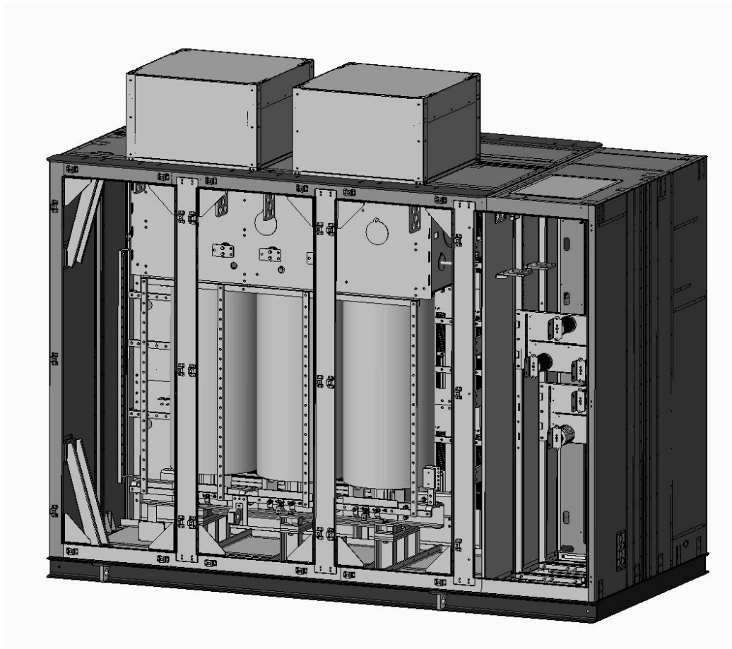
图3.17 变压器副边结构图
