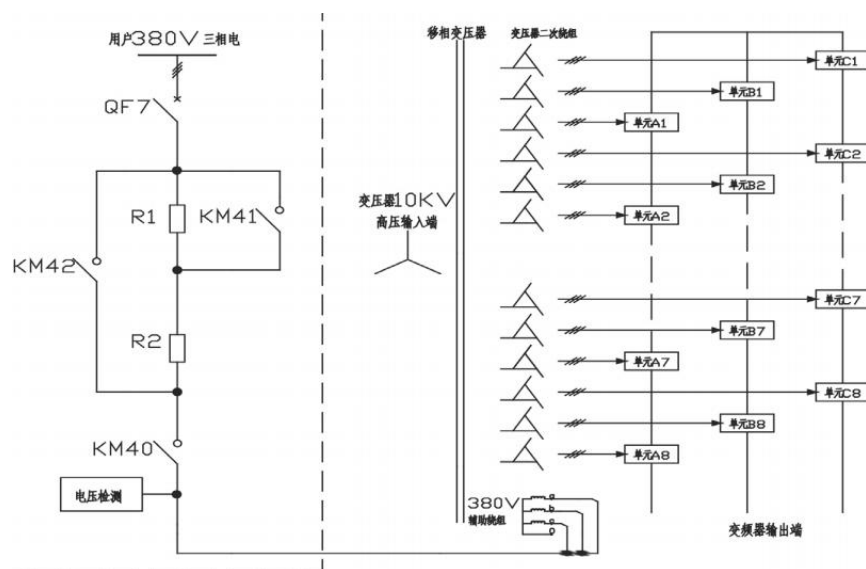
图3.21 预充电箱一次回路
