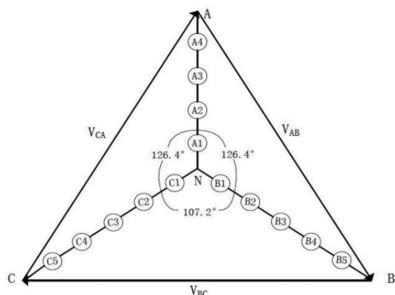
图6.7 中性点漂移输出示意图
