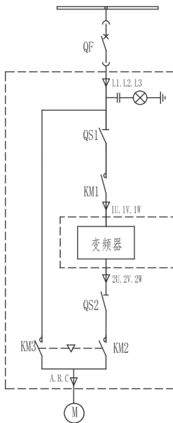
图3.24 自动旁路柜一次图
