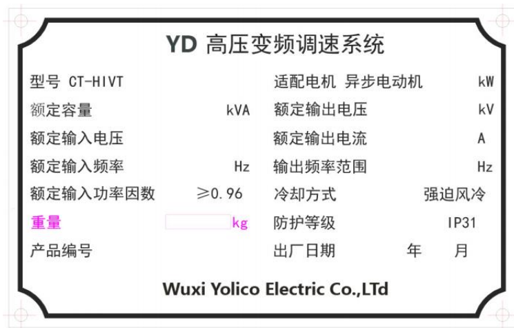
图2.1 产品铭牌信息
