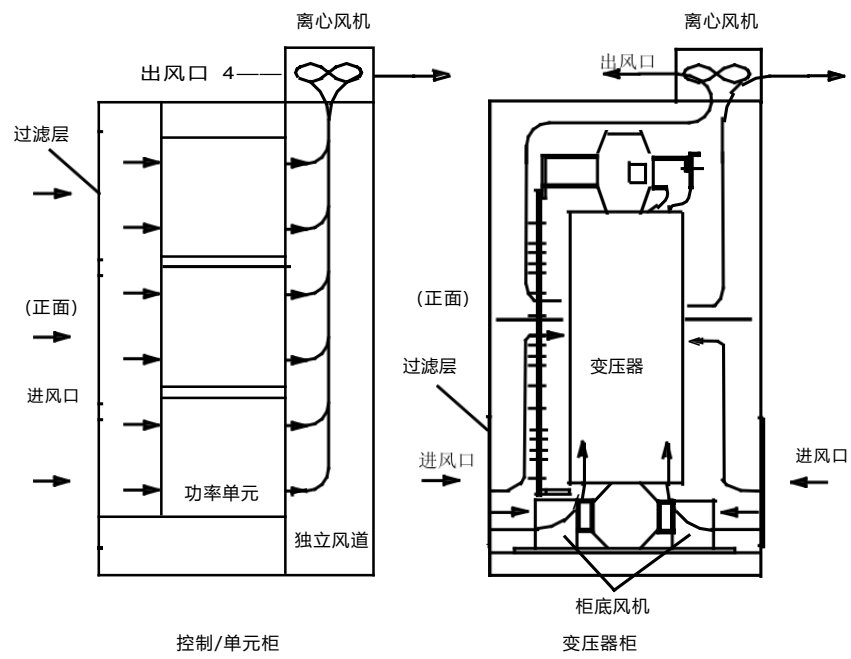
图7.3 6kV通用变频冷却风路图
