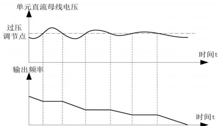
图6.4 过压调节示意图
