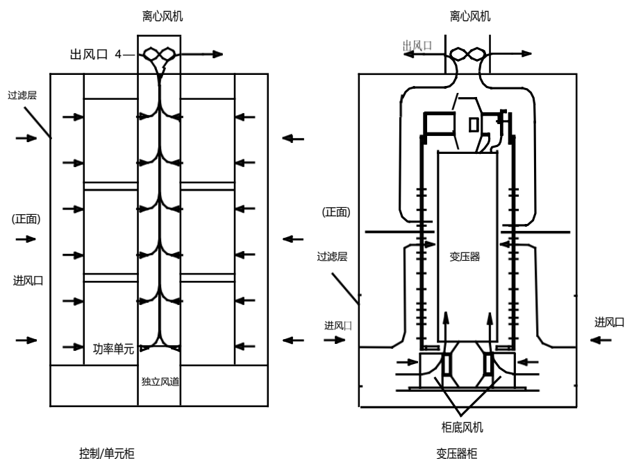
图7.4 10kV通用变频冷却风路图
