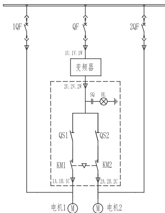
图3.26 自动切换柜一次图
