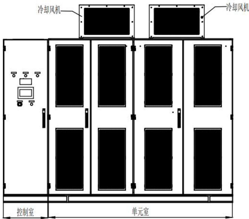
图3.14 变频器一体柜
