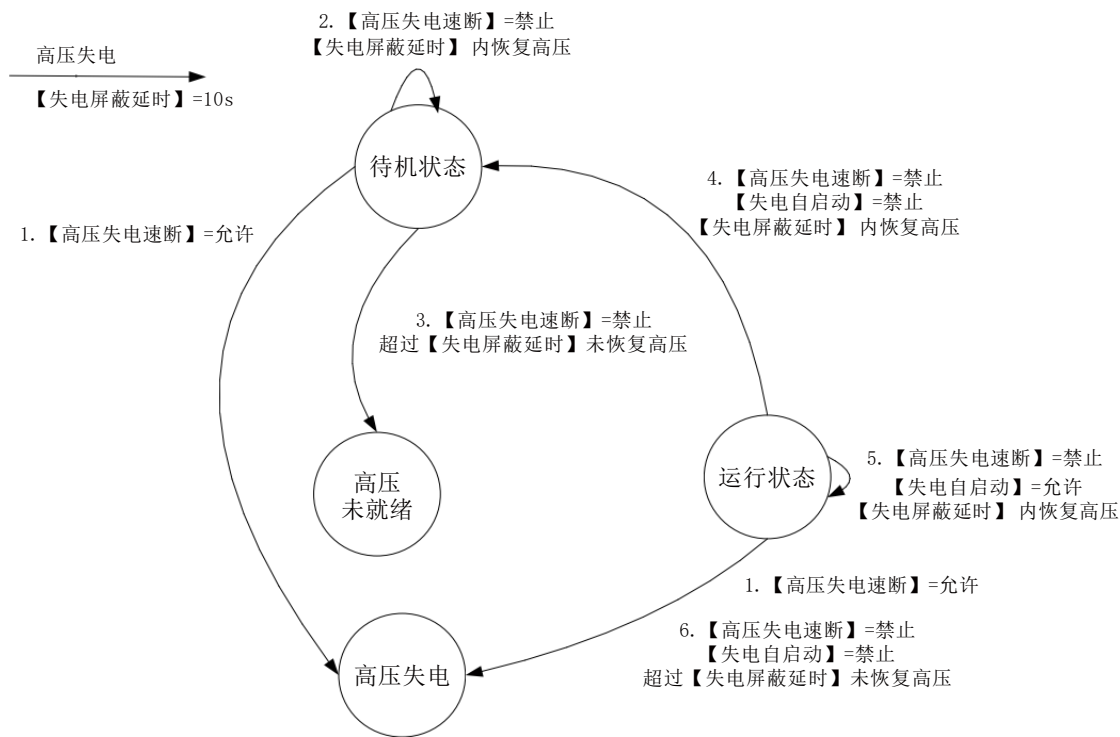
图6.1 高压失电状态机
