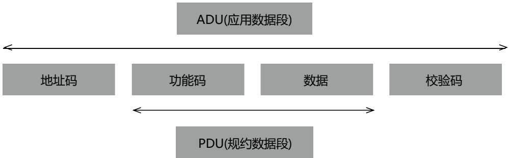
图11.2 数据包结构
