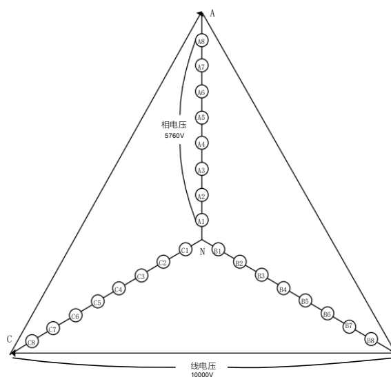
图3.4 10kV变频器单元电压叠加图
