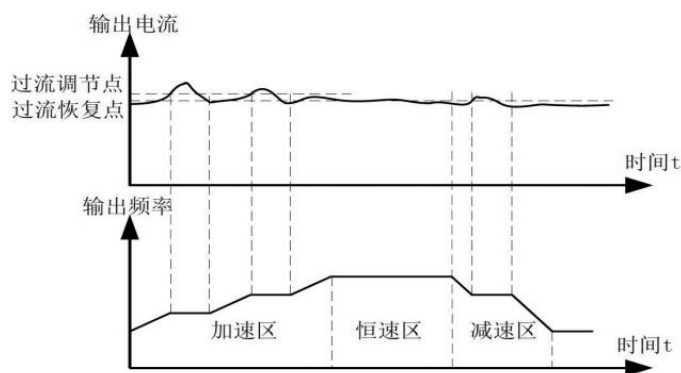
图6.3 过流调节示意图
