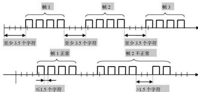
图11.1 数据及帧格式
