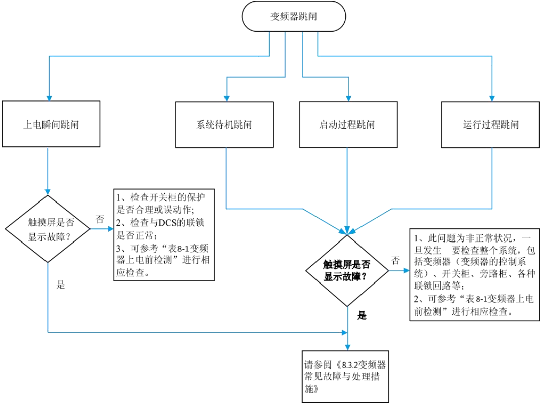
图8.1 变频器跳闸检测流程图
