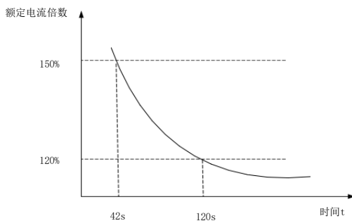
图6.2 反时限保护示意图
