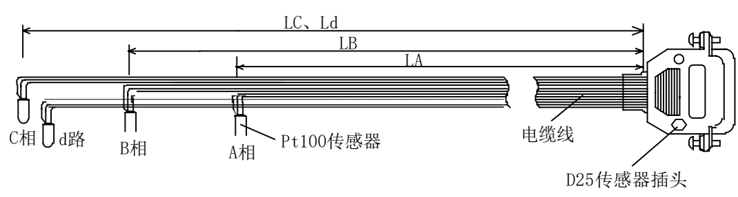
G/I型四路电缆连接示意图
