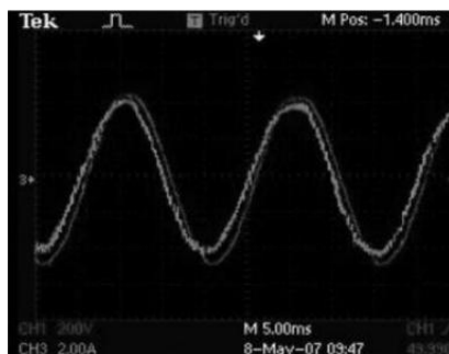
图2.2 30脉冲输入波形（CH1电压、CH3电流）
