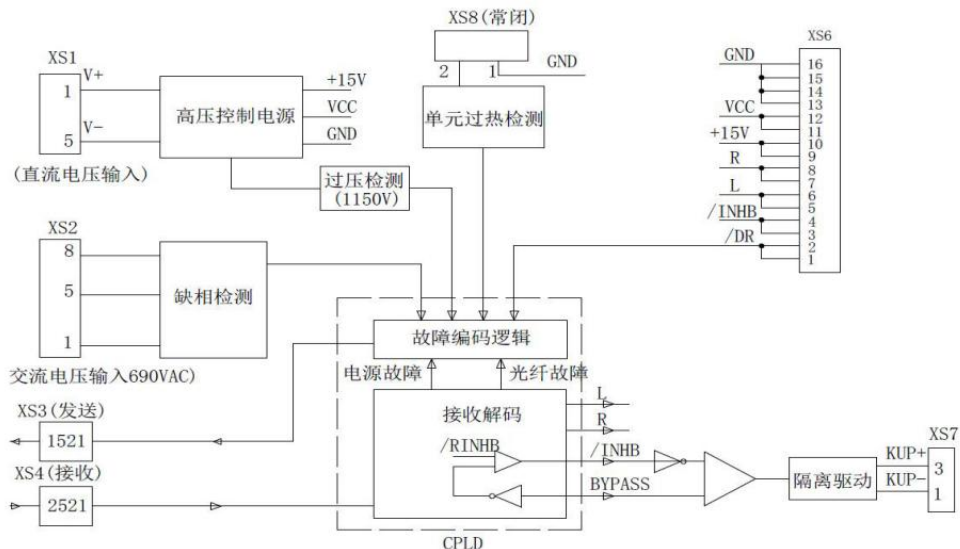
图3.10 单元控制板原理图
