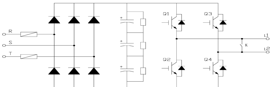
图3.9 功率单元拓扑图
