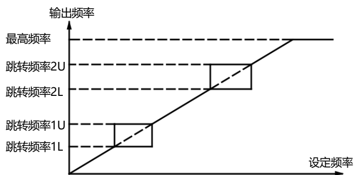
图5.24 跳转频率
