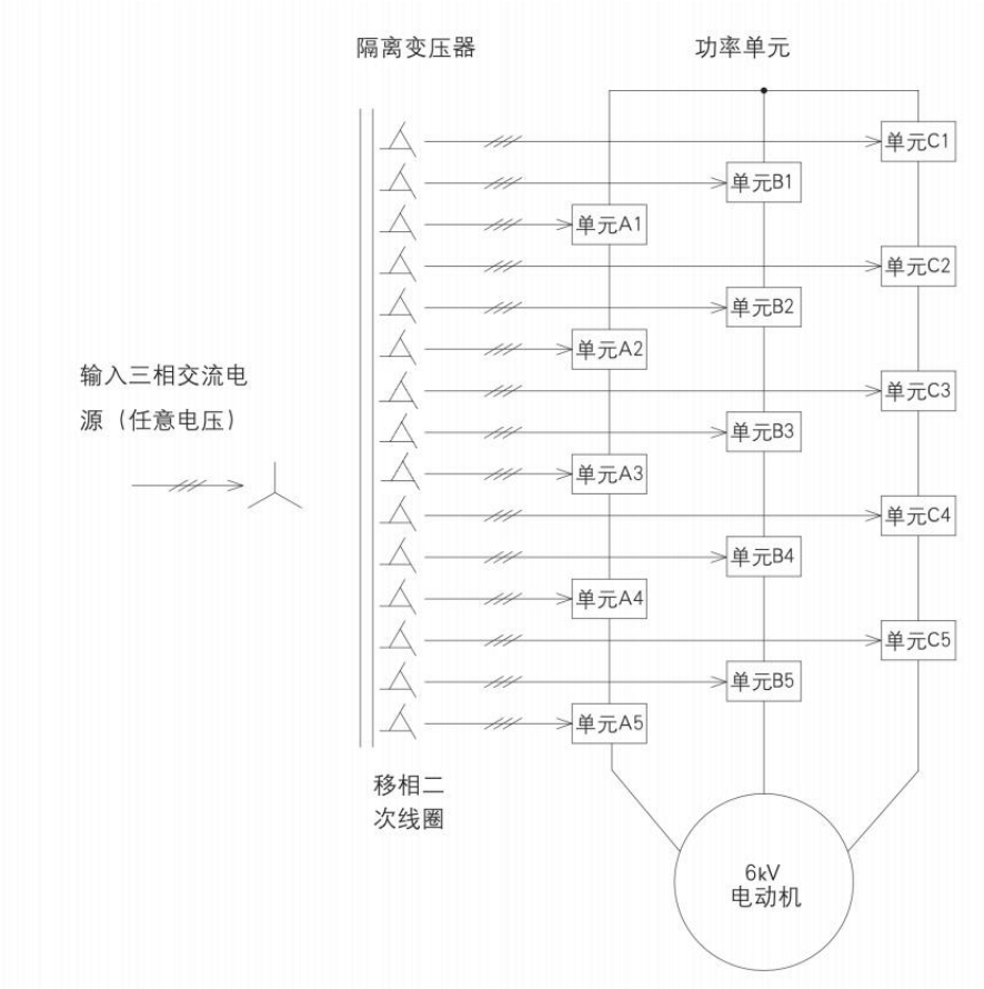
图3.2 变频器主回路图（6kV为例）
