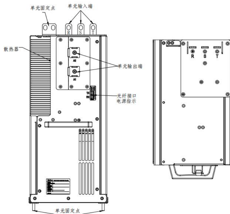
图3.12 功率单元外形图
