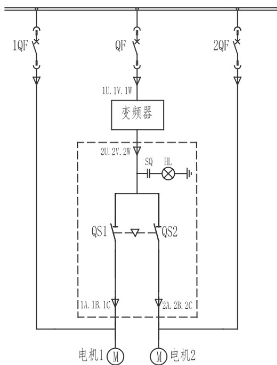
图3.25 手动切换柜一次图
