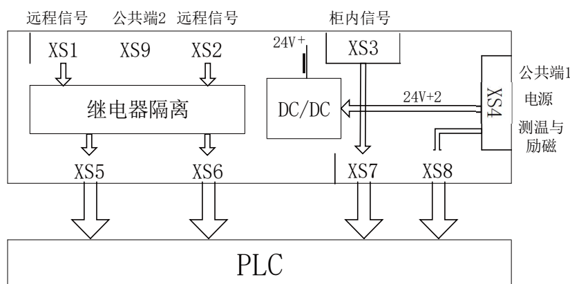
图3.8 接口上板原理框图
