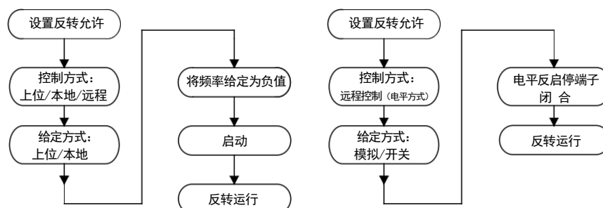
图5.21 反转运行流程图
