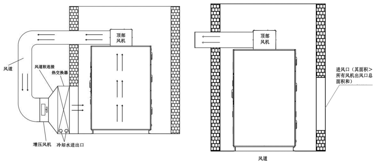
图7.5 空水冷图
