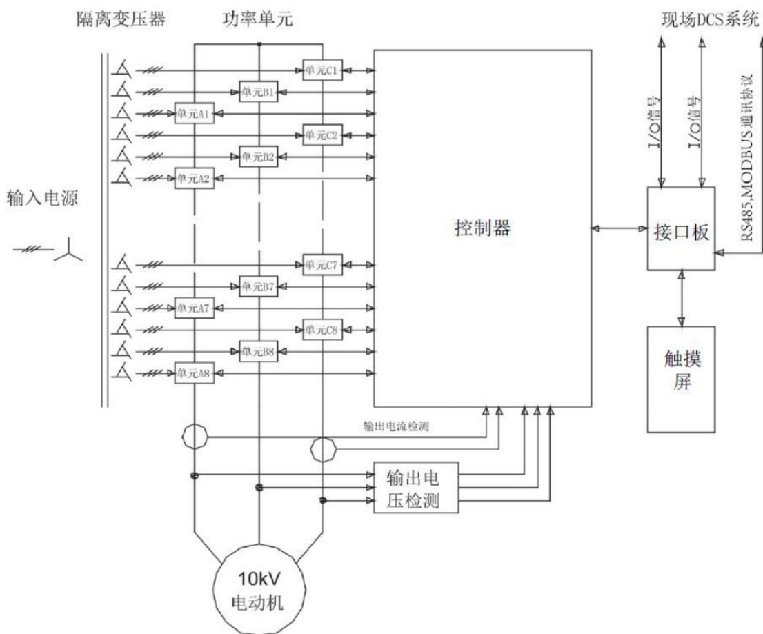
图3.1 变频器系统图 (10KV为例)
