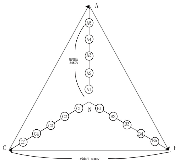
图3.3 6kV变频器单元电压叠加图
